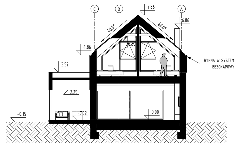
PRZEKRÓJ PRZEZ SALON
